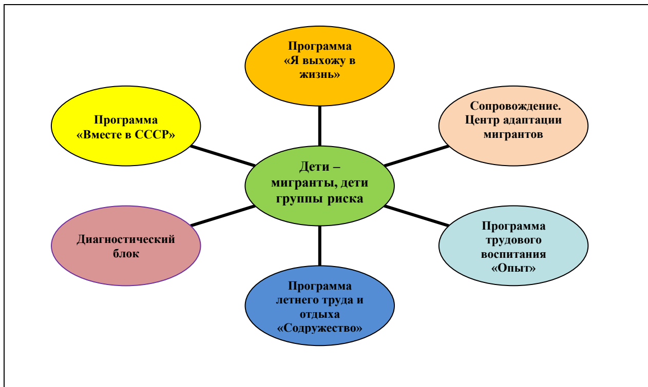
Рисунок 2. Содержание Программы
